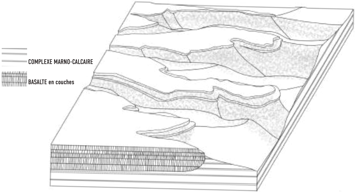
BLOC GÉO-MORPHOLOGIQUE DU COIRON ACTUEL
