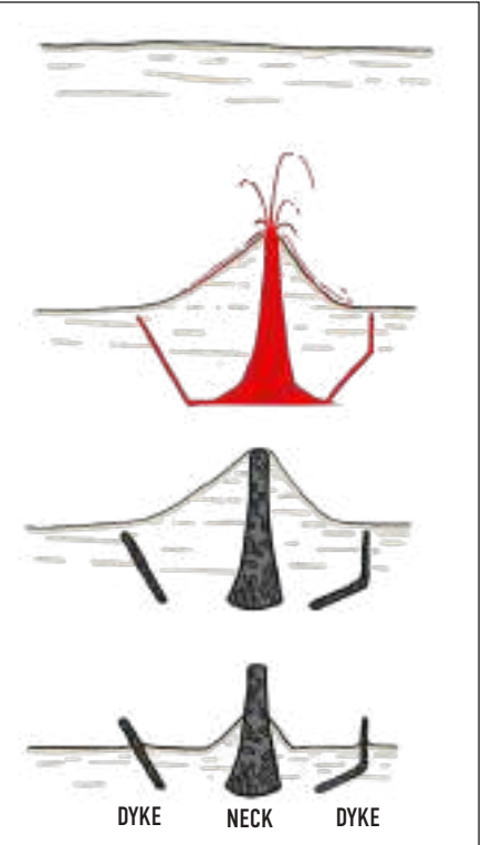
SCHÉMA DE LA FORMATION DES NECKS ET DYKES VOLCANIQUES
